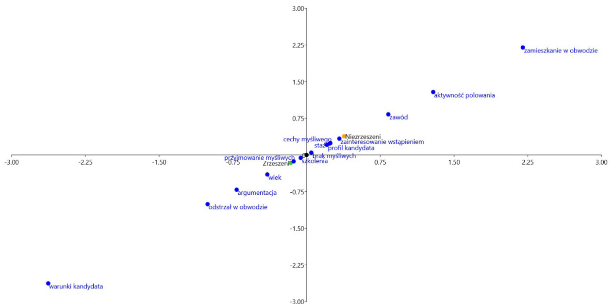
Rys. 5. Analiza korespondencji (CA) dla grup myśliwych zrzeszonych i niezrzeszonych. Wartości własne dla osi 1\lambda = 0,61 (100,0%), dla osi 2\lambda < 0,001 (<0,001%)
